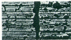
800fache Vergrößerung eines normalen Ferrit-Kopfes nach gleicher Betriebsdauer
