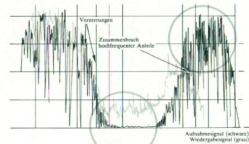
Abhängigkeit der dynamischen Verzerrung ohne AKAI A.D.R.-System
