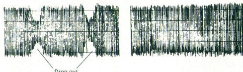
Einfach-Capstan-Antrieb. Amplitudenschwankungen durch mangelnde Bandführung
