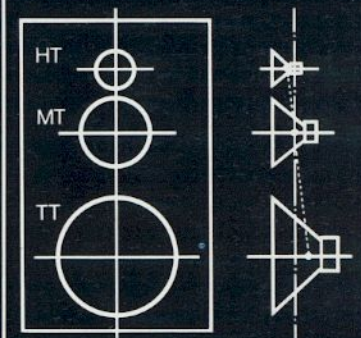
Fig. 2 IN-LINE Arrangement Lautsprecher in einer Linie.
