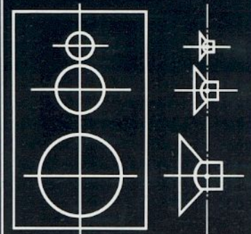
Fig. 1 PLUMB-IN-LINE Arrangement Schallzentrum jedes Lautsprechers auf einer Senkrechten.
